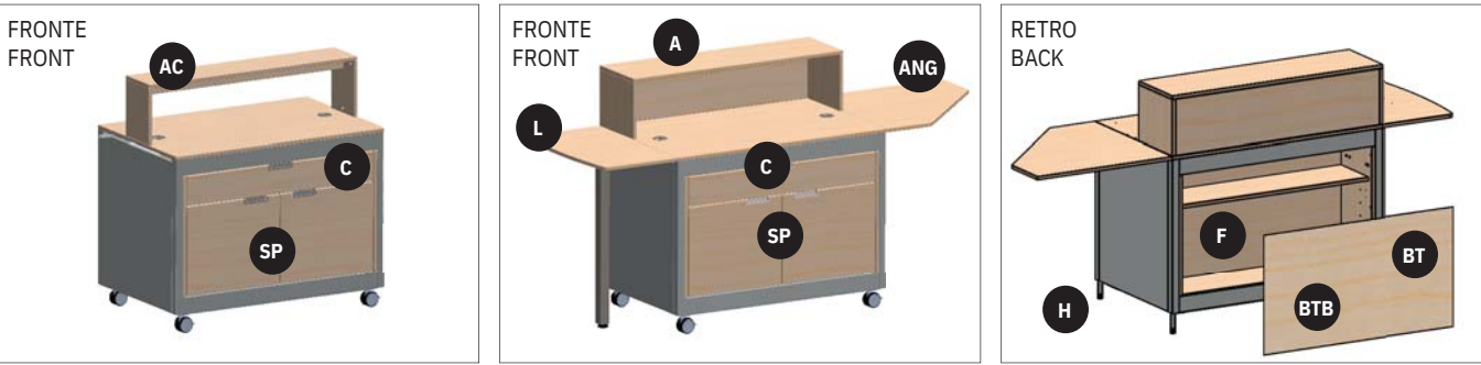
MODULO PER COSTRUZIONI SU MISURA CUSTOMIZED CONNECTION MODULE Spesso gli spazi disponibili non sono perfettamente compatibili con le dimensioni standard del Break. Nel caso, Opt. L e Opt. ANG possono essere personalizzati/modificati in base ai tuoi bisogni. Often the spaces available are not perfectly compatible with the standard dimensions of the Break. In case, Opt.L and Opt.ANG can be customized / modified according to your needs.
